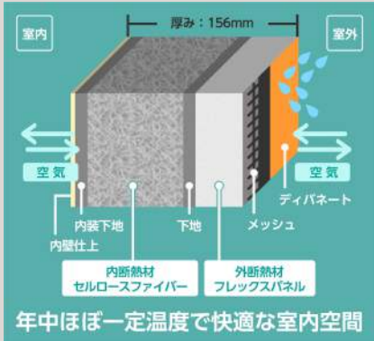
内断熱材セルロースファイバー+外断熱材フレックスパネル
